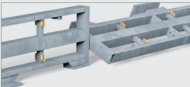
Kipplängenbegrenzer (KLB)
